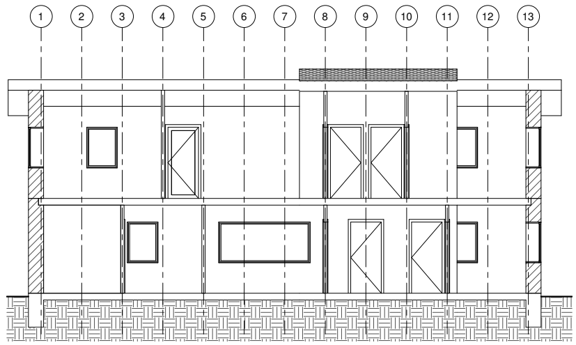
6 Længdesnit 1:50
