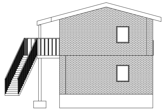
4 Gavl øst 1:50
